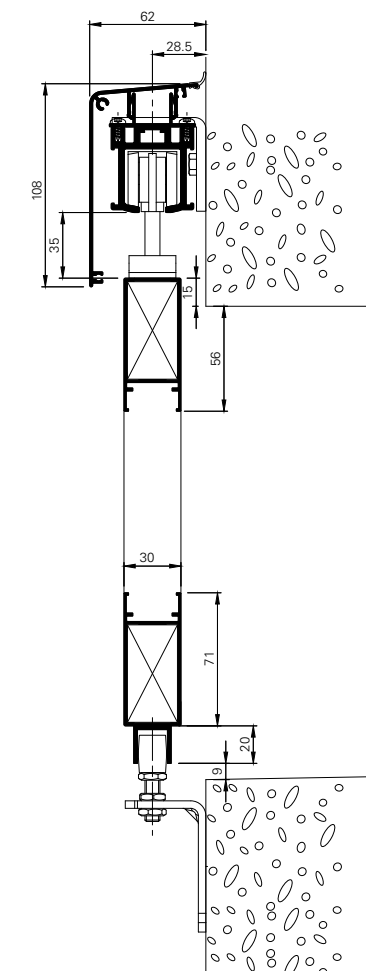
Coupe verticale
